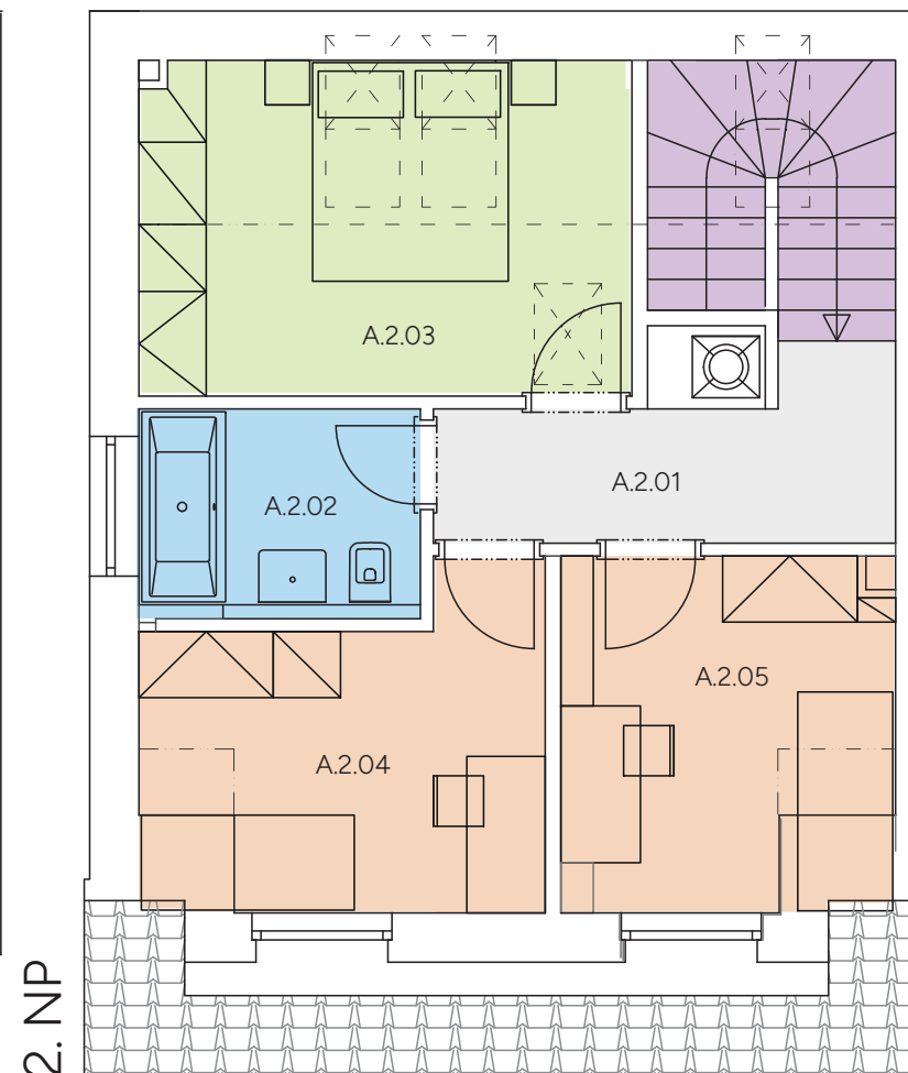
TABULKA MÍSTNOSTÍ 2.NP
